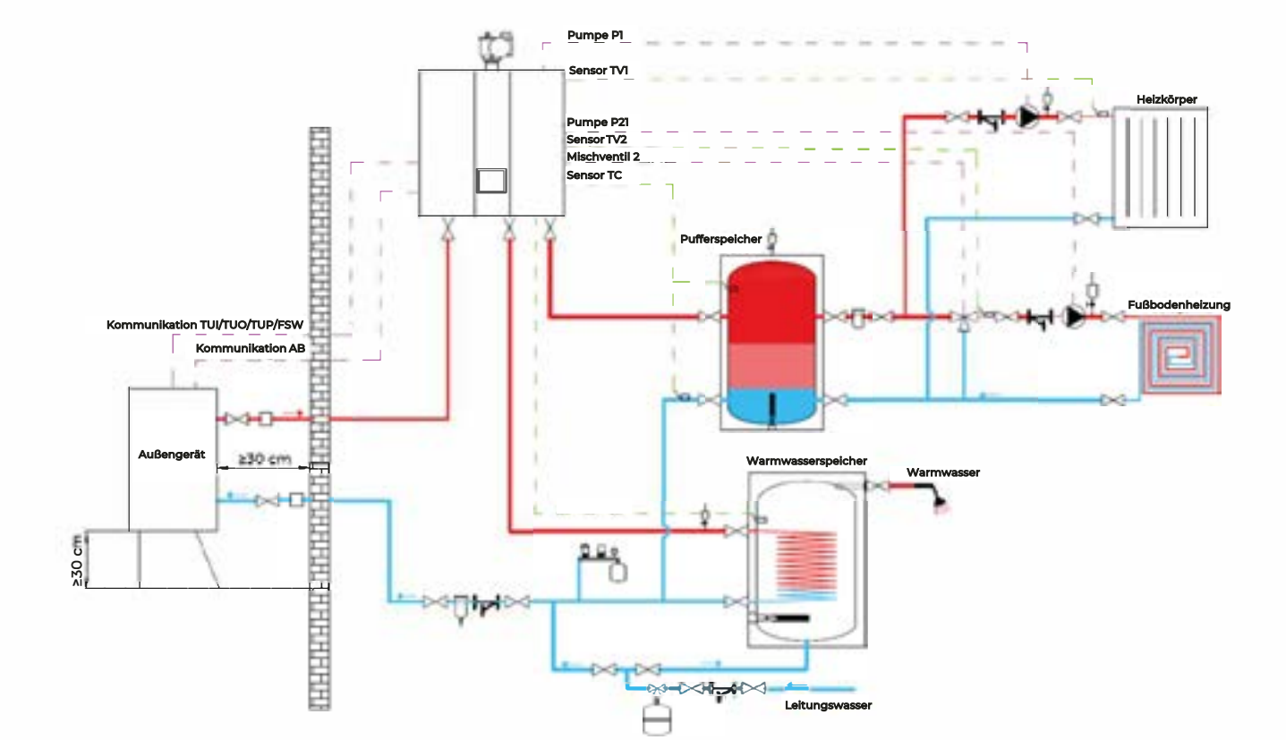
Schaltplan: THERMAL 6/9/12/15/19 kW mit kombinierter Heizung + Warmwasser
